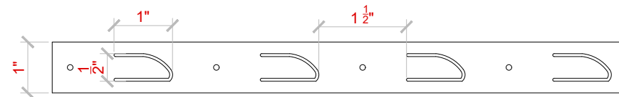
BAFFLE
